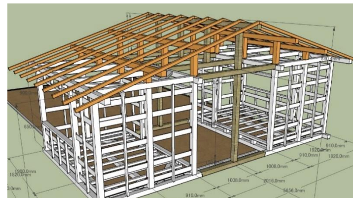
※木造軸組2/3模型
